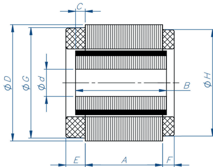
FRAMELESS MOTOR SIZE DATA &amp; PARAMETERS [mm]
