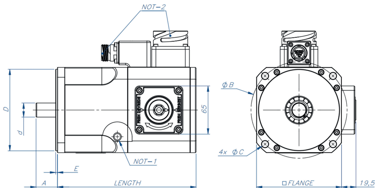
SERVO MOTOR SIZE PARAMETERS [mm]
